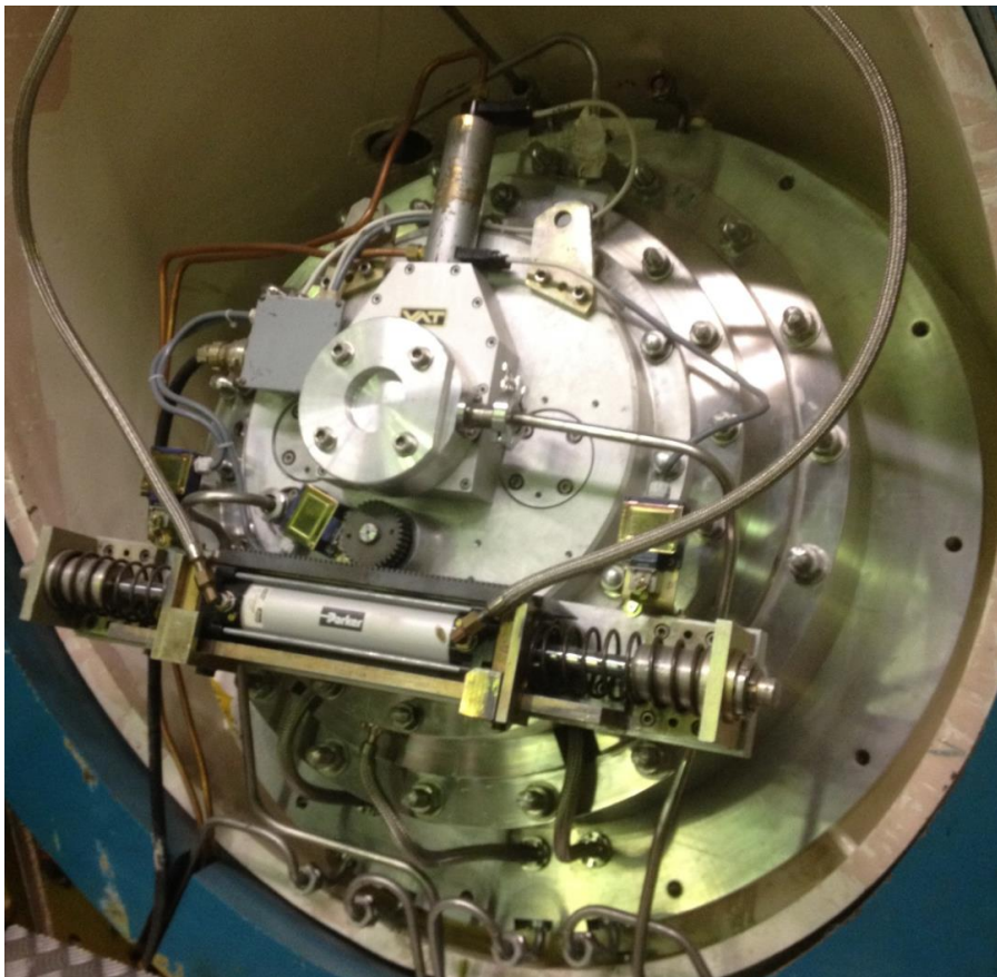
Photo : vue du bridage arrière du doigt de gant IH3 avant remontage de l'instrument
