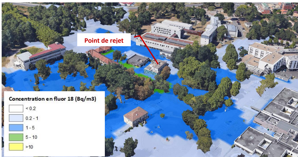
Figure 24 : vues 3D des concentrations au sol en moyenne annuelle en fluor 18 en Bq/m 3
