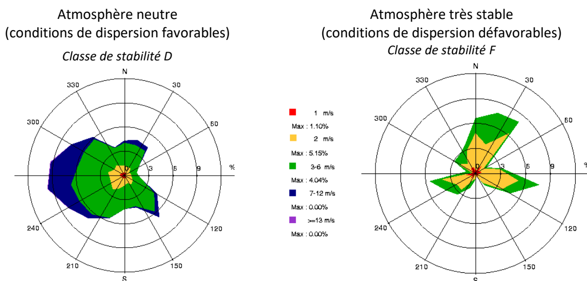
Figure 14 : roses des vents par classe de stabilité
