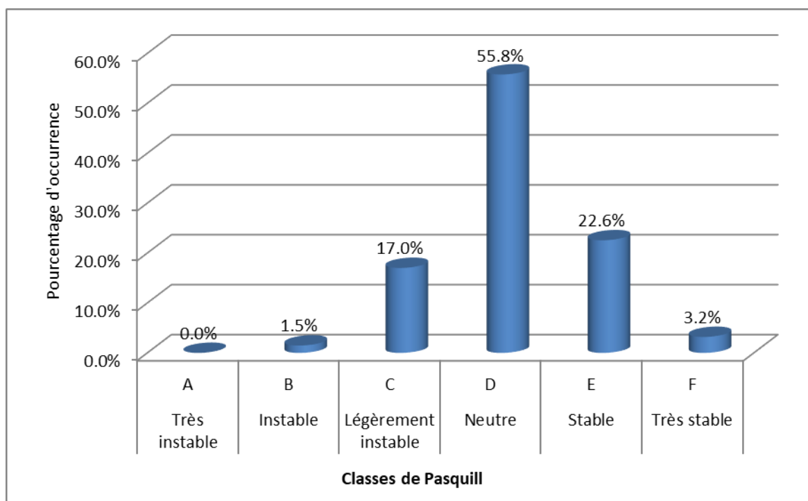
Figure 13 : répartition des observations en fonction de la stabilité atmosphérique
