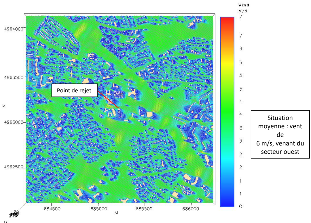
Figure 20 : lignes de courant et vitesse du vent à 2m au-dessus du sol
