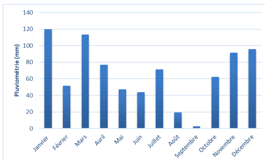
Figure 16 : variation de la pluviométrie sur l'année (période du 01/01/2018 au 31/12/2018)
