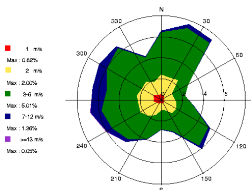
Figure 18 : rose des vents calculée à partir des échéances sans pluie
