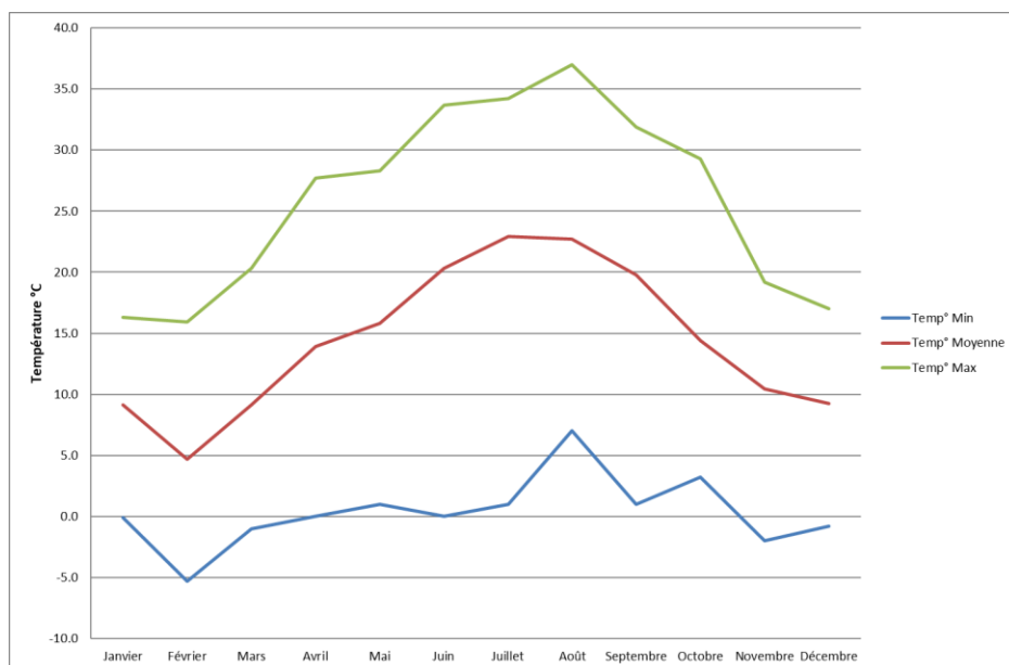
Figure 15 : variation de la température sur l'année (période du 01/01/2018 au 31/12/2018)
