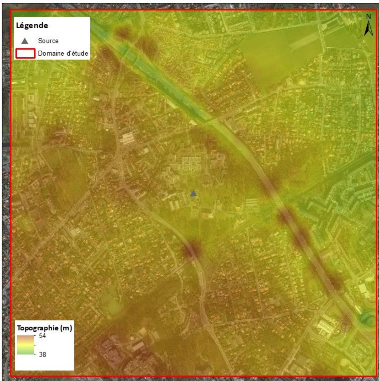
Figure 10 : topographie du domaine d'étude
