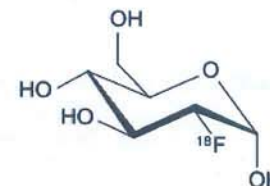
Figure 1 : Structure chimique du 18FDG
