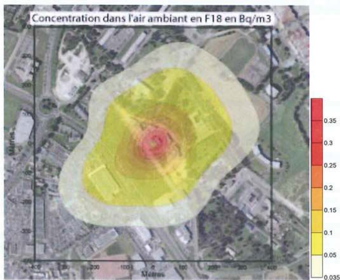
Figure 11 : cartographie des concentrations en Fluor 18 dans l'air dans l'environnement du site
