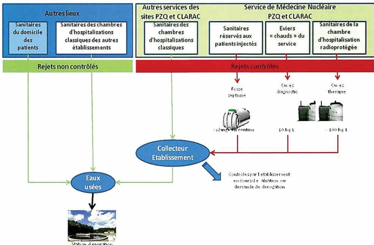
Figure 3 : Gestion des effluents liquides contaminés par des radionucléides de période < 100 jours générés par le service de Médecine Nucléaire.
