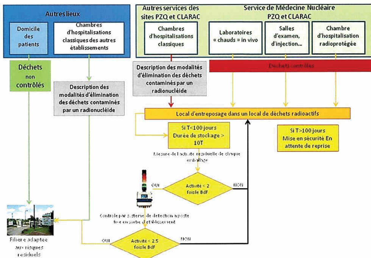
Figure 4 : Gestion des déchets contaminés par des radionucléides générés par les activités de médecine nucléaire.
