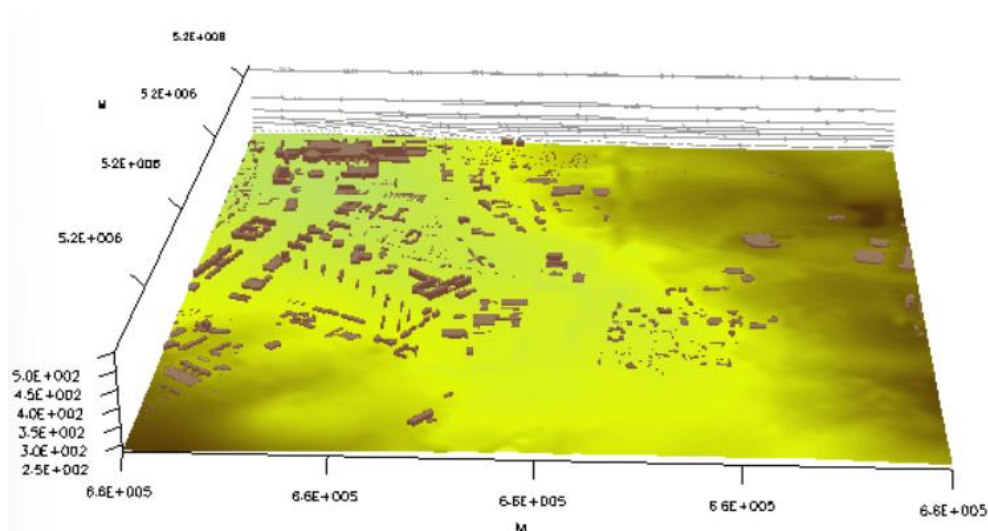
Figure 17 : boîte de calcul
