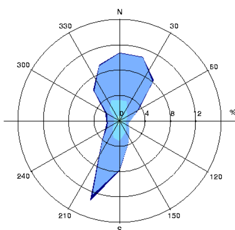
Figure 7 : rose des vents générale – 2022
