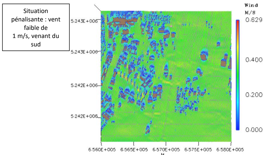
Figure 16 : lignes de courant et vitesse du vent à 2 m au-dessus du sol
